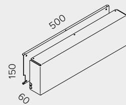
095-910 Carter Steuerung/Netzteil
