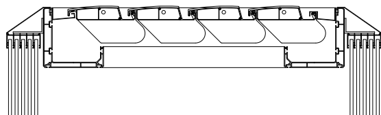
Rotation der Lamellen um 90°
