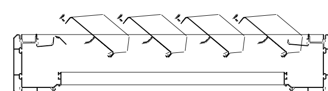
Rotation der Lamellen um 140°
