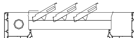
Rotation der Lamellen um 69°
