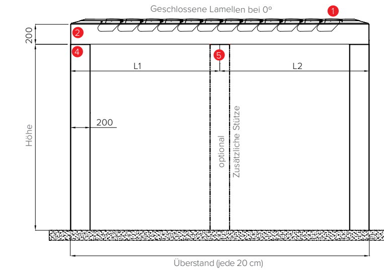
Seitenansicht
