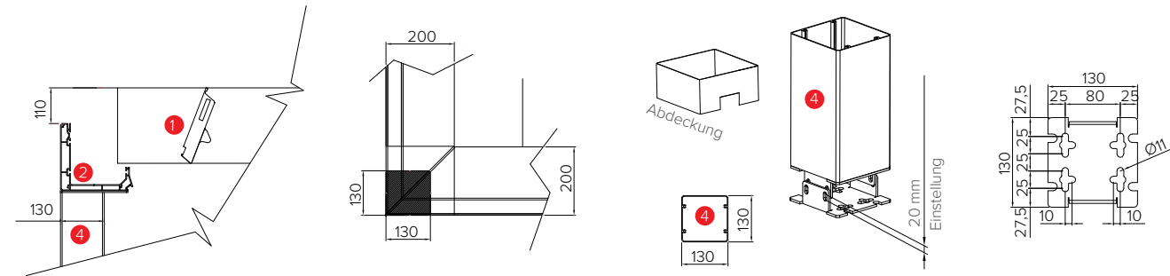
Aussparung zum Einsetzen von LED-Leuchten
