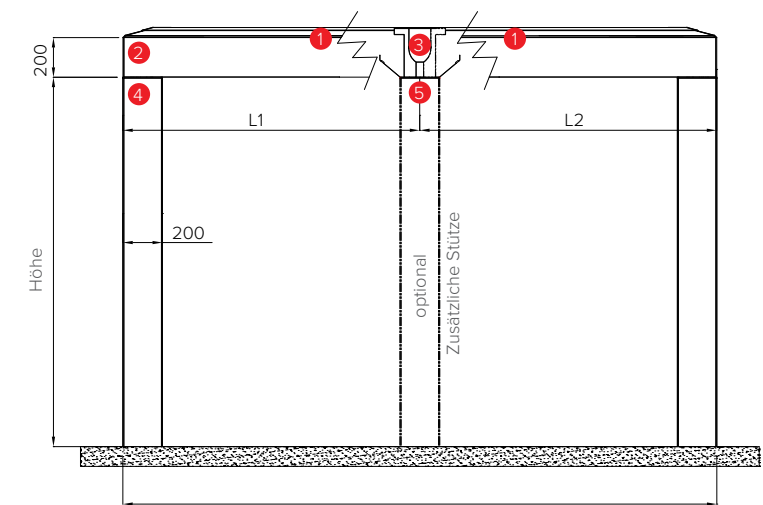
Seitenansicht
