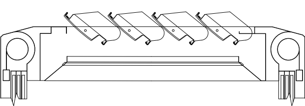
Rotation der Lamellen um 140°
