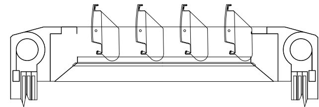
Rotation der Lamellen um 90°
