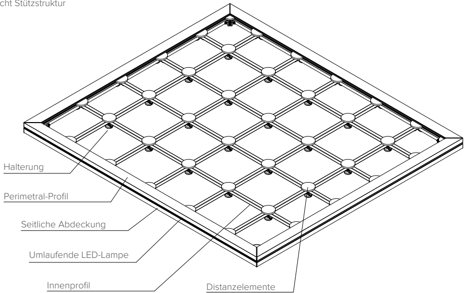
Ansicht Stützstruktur
