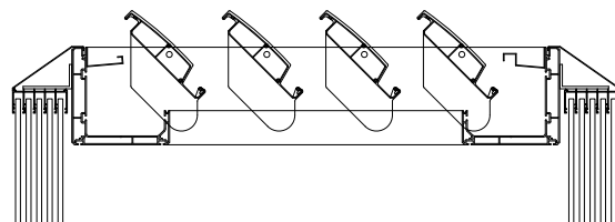
Rotation der Lamellen um 140°
