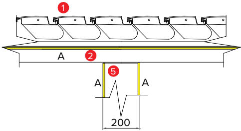
Seitenansicht
