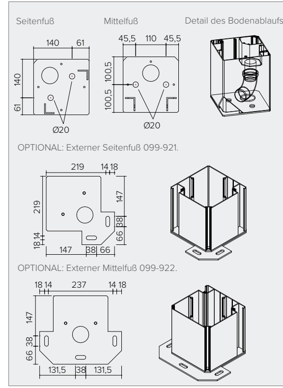
Gehäuse für Steuergeräte. 081-924
