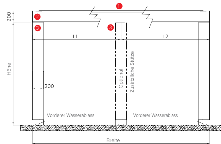
Vorderansicht
