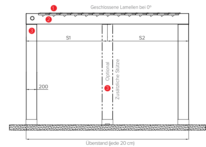
Seitenansicht
