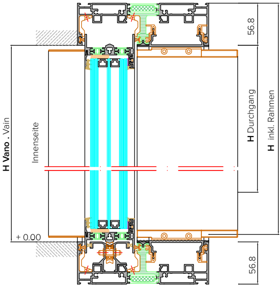
Außenansicht
